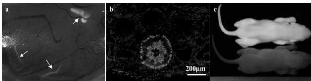
図. MT- myc ラット精巣への精子幹細胞移植. (a) ドナー細胞移植 3 ヶ月後の精巣. EGFP 発現コロニー (矢印)、(b) ドナー細胞由来の EGFP を発現する精細管断面. 基
