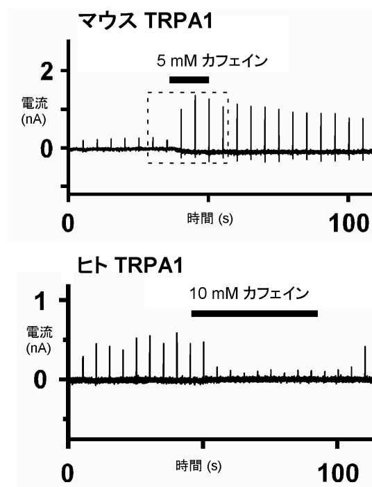
図 1. 遺伝子導入した HEK293 細胞のパッチクランプ法による記録。膜電位固定下で、ランプ波形の電位刺激を繰り返して与え、電流応答を記録した。(上) マウス TRPA1 チャネルを発現させた細胞からの記録。5 mM カフェインの投与により、チャネル電流が増加した。(下) ヒト TRPA1 チャネルを発現させた細胞からの記録。10 mM カフェインの投与により、チャネル電流が減少した。
