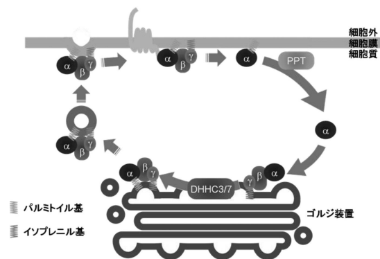
図 1. パルミトイル化を介した G\alpha 細胞内動態モデル 細胞膜上の G\alpha は脱パルミトイル化されて細胞質に移行し、ゴルジ装置に存在する DHHC3 および DHHC7 により再パルミトイル化され一時的にゴルジ装置に集積する。 G\alpha はその後 G\beta\gamma とともに小胞輸送などにより細胞膜に移行する。PPT: 脱パルミトイル化酵素。
