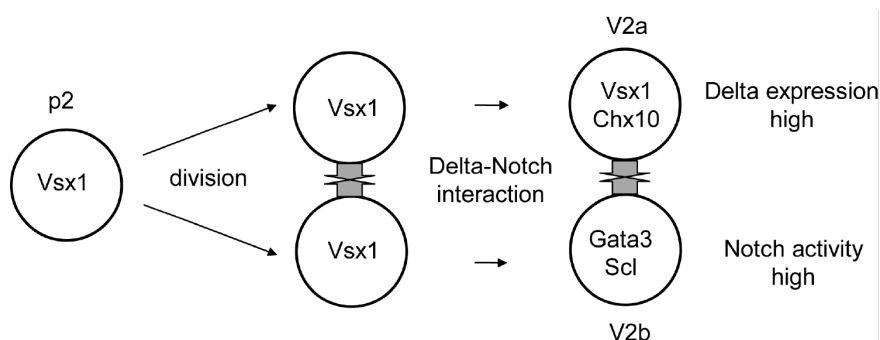
図 1. V2 ニューロン分化の模式図
