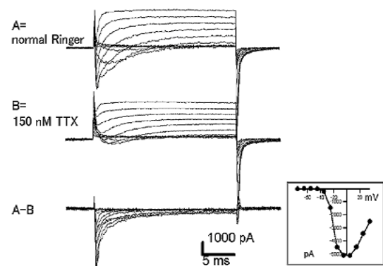
図2 ラット小脳プルキンエ細胞の細胞体から単離した Outside-out patch による電位依存性 Na チャンネル電流の記録。TTX をかける前後で引き算を行い、Na チャンネルを流れる電流のみを得ることができる。
