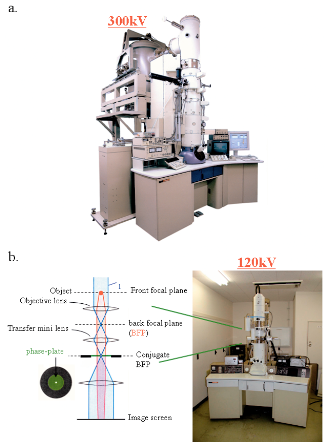
図2. 2つの電子位相顕微鏡装置
