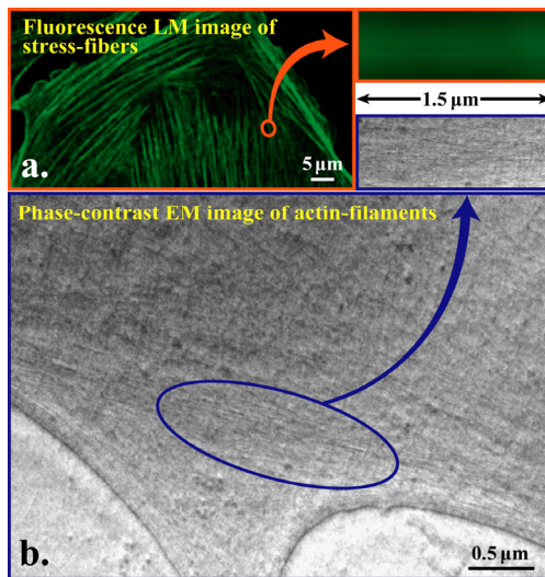
図4. 細胞 (PtK2) 内のアクチン繊維の光顕と電顕の解像度比較。 a. ファロイジンで染色したストレスファイバーの蛍光顕像。 b. ストレスファイバー内のアクチン繊維を解像する 300kV ヒルベルト微分像。
