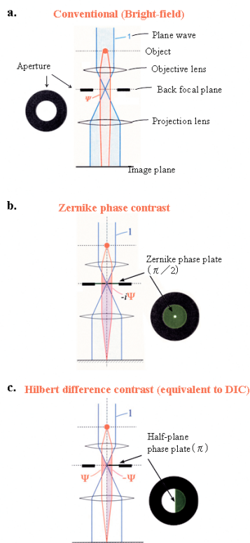
図1. 電子位相顕微鏡法の3種 a. 焦点はずし(デフォーカス)を導入し、分解能を犠牲にしてコントラストを向上する通常法(明視野法)。
