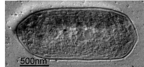
図3. シアノバクテリアの 300kV 全細胞氷包埋像と 100kV プラスチック包埋切片像。
