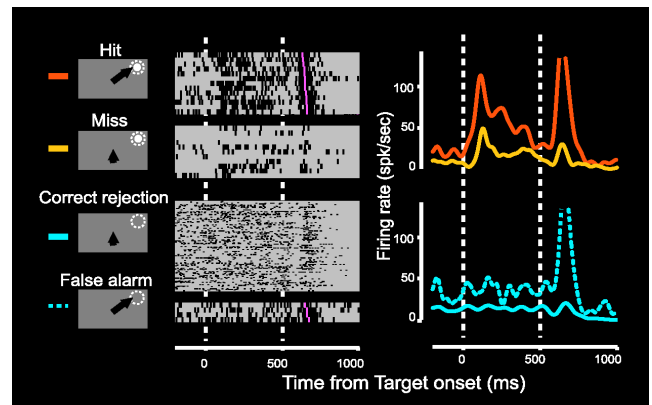
図2 片側一次視覚野除去後のサルから計測された、視覚刺激検出課題遂行中の損傷側上丘の神経活動。損傷側上丘・中間層の神経細胞ではサルの行動と関連した視覚応答の変化が見られる。ターゲットの検出・サッケードによる定位に成功した試行 (Hit trial) では明確な視覚応答が観察されるのに対し、サルがターゲットを検出できなかった試行 (Miss trial) では、視覚刺激はまったく同じであるにもかかわらず視覚応答は減衰している。
