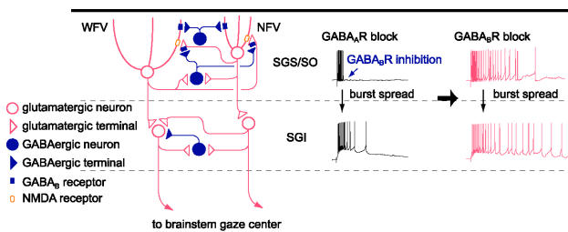
図1 上丘での GABA B 受容体を介したバースト発火の制御機構の模式図。GABA B 受容体は上丘浅層の narrow field vertical cell (NFV) と wide field vertical cell (WFV) のシナプス後膜およびグルタミン酸作動性神経終末に発現している。浅層の GABA 作動性ニューロンのバースト発火によって遊離された GABA が、これらの受容体に作用すると NFV では過分極が、WFV ではシャunting抑制が誘発され、また、シナプス終末からのグルタミン酸遊離が抑制される。
