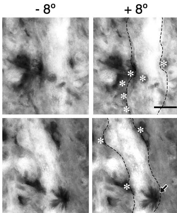
図 1; 超高压電子顕微鏡のステレオペア像（±8° の傾斜をかけて撮影）。放射状沈着物として観察されている TMB 産物（矢印）で、逆行性標識された SNB ニューロンの樹状突起（破線）に終末する GRP ニューロンの軸索（*）。Bar = 2 μm.
