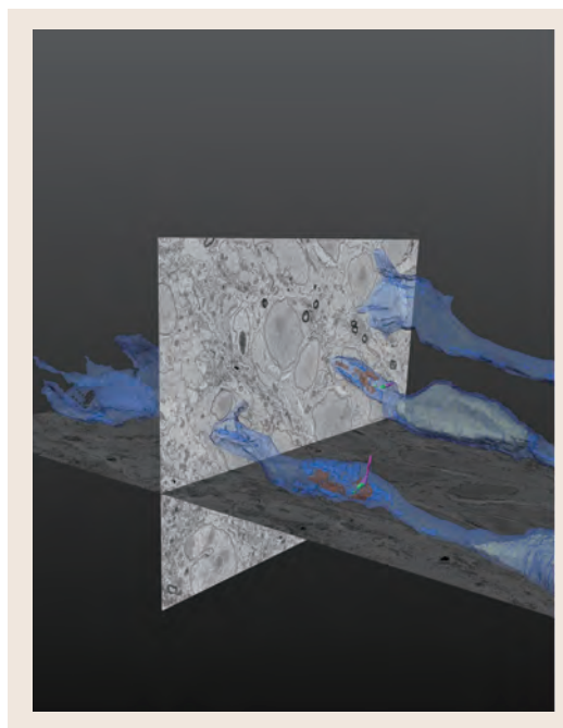
図2 成体マウスの脳内を移動する新生ニューロンの微細形態を、生理研の連続ブロック表面走査型電子顕微鏡によって観察した。哺乳類の脳室下帯では継続的に神経幹細胞からニューロンが産生され、鎖状の細胞塊を形成しながら嗅球へ移動する。各々のニューロンには、基底小体（緑）、一次繊毛（ピンク）、核（黄）、ゴルジ体（オレンジ）、ミトコンドリア（青）などの構造物が観察される (Matsumoto et al., J Neurosci 2019)。
