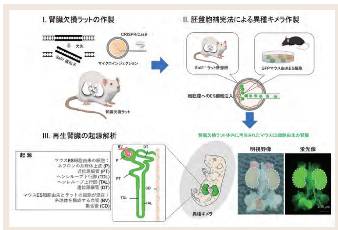
図1. 異種胚盤胞補完法による腎臓再生モデル. I. ラット体内にマウスの腎臓を再生させるため、ゲノム編集技術を使ってラット自身の腎臓を欠損させたラットをまず作製する. II. 腎臓欠損となる運命にある胚盤胞期受精卵に GFP マウス由来 ES 細胞を顕微注射して仮親ラットに移植すれば、生まれてきた異種キメラの体内には ES 細胞由来の腎臓が作られている. III. 再生された腎臓を組織学的に解析したところ、糸球体や尿細管など、ネフロンのほとんどの組織が GFP 陽性の細胞から構成されていた。
