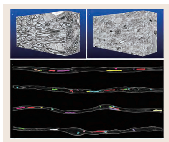
図1 コントロール (a) と脱髄モデルマウス (b) の脳組織の連続電子顕微鏡画像の再構築像と、軸索のミトコンドリアの 3 次元再構築像 (c). Ohno et al. PNAS (2014) より修正・転載
