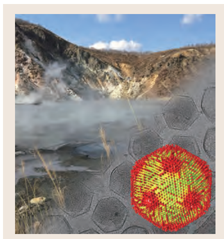
図2 クライオ電子顕微鏡により明らかになったメドゥーサウイルスの構造。メドゥーサウイルスは日本の温泉水から発見された (背景写真)、進化上最も真核生物に近いウイルスである (Yoshikawa et al. 2019)
