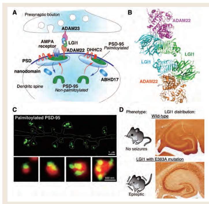
図 (A) 独自に発見した AMPA 受容体制御分子：パルミトイル化酵素 DHH2、脱パルミトイル化酵素 ABHD17 とてんかん関連リガンド・受容体 LGI1・ADAM22、そして、パルミトイル化 PSD-95 で構成されるナノドメイン。(B) LGI1・ADAM22 複合体の X 線結晶構造。(C) パルミトイル化 PSD-95 特異的プローブと超解像顕微鏡によるポストシナプスナノドメインの発見。(D) 家族性てんかんのモデルマウスの作成と解析：LGI1 E383A 変異体蛋白質は、蛋白質構造異常によって小胞体に留まり、分泌が低下し、ADAM22 受容体との結合量が低下する。
