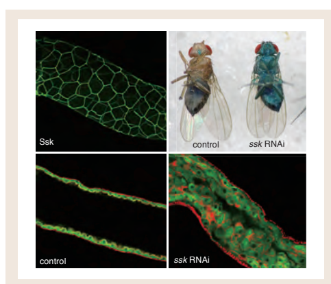
ショウジョウバエの腸管における細胞間結合スモースセプテートジャンクションの機能
