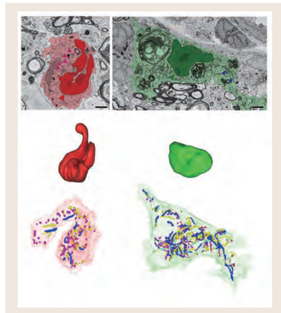
図2 マウス脱髄モデルにおける単球由来 (赤) とミクログリア由来 (緑) のマクロファージの電顕画像 (上段) および核 (中段) とミトコンドリア (下段) の 3 次元再構築像。Katoh et al. Sci Rep (2017) より修正・転載
