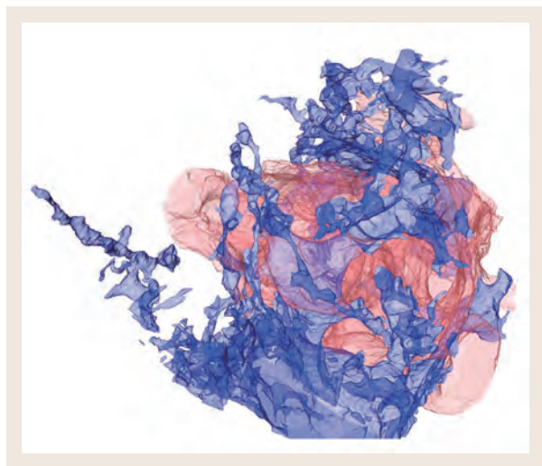
図1 生理研に設置されている連続ブロック表面走査型電子顕微鏡（SBF-SEM）により、脳梗塞で活性化して増殖・肥大化するアストロサイト（青色）と呼ばれる細胞が、再生したニューロン（赤色）の移動を妨げている様子を三次元的に観察した (Kaneko et al., Sci. Adv. 2018)。
