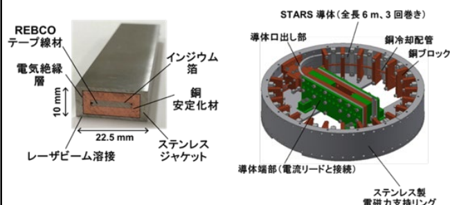
高温超伝導STARS導体（断面図とコイル形状試験体（直径60cm））
