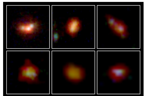
ジェイムズ・ウェッブ宇宙望遠鏡の近赤外線分光器で得られた131億年から133億年前の6個の銀河の画像（クレジット：NASA, ESA, CSA, K. Nakajima et al.）
