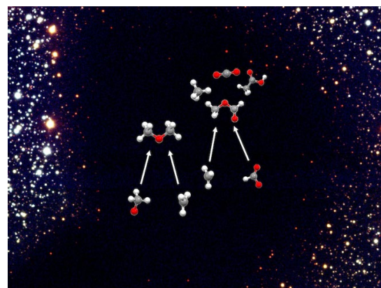
低温の星形成領域内で複雑有機分子（ジメチルエーテル、ギ酸メチル）ができる反応経路のイメージ。(クレジット：ABC、背景画像：ESO)
