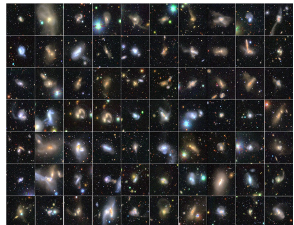
すばる望遠鏡に搭載した超広視野主焦点カメラHyper Suprime-Cam (ハイパー・シュプリーム・カム) で取得した画像から選ばれた激しい衝突・合体の現場にある銀河。大きく形が崩れた銀河が多く、合体の激しさが見て取れます。（クレジット：国立天文台）
