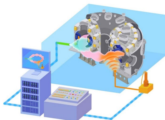
計算機上に再現した仮想プラズマを通して現実のLHDプラズマを制御するデジタルツイン制御のイメージ図
