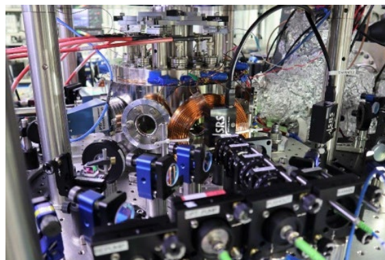
冷却原子（中性原子）方式量子コンピュータの研究開発
