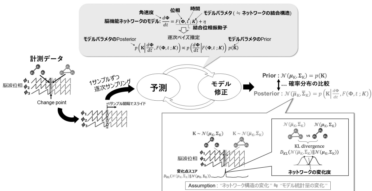
図18 位相同期ネットワーク構造の変化点推定手法の概念図 脳波等の計測データに対して結合振動子モデルでの逐次的予測データのフィッティングを行うことで位相同期ネットワーク構造の時間的な変化様相を推定する。
