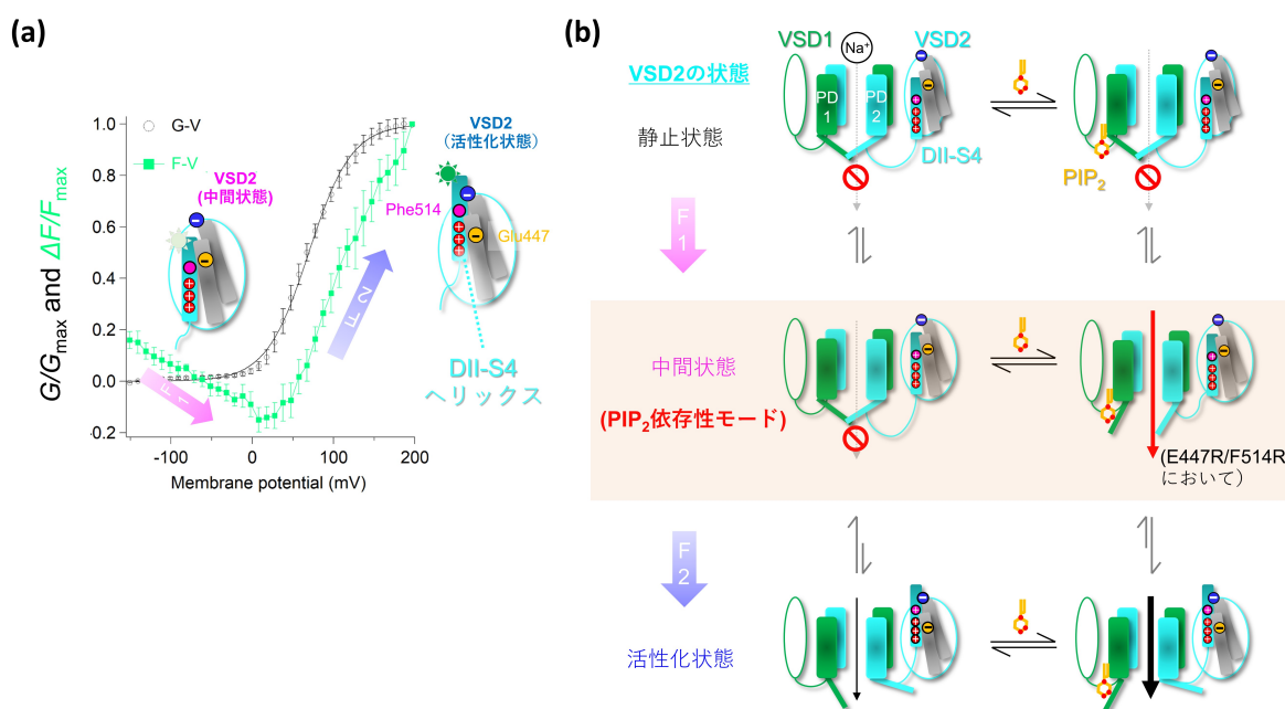
図1 TPC3のDII-S4は中間状態をとる。(a)TPC3における膜電位固定下蛍光測定法の結果。電流(○)が生じない過分極側でDII-S4の動きを反映する蛍光(■)は減少(F1)し、脱分極側では増加(F2)する。F1に対応する動きにより、DII-S4は中間状態に遷移する。(b)2番目のVSD(VSD2)の構造変化に依存したチャネルの状態遷移のスキーム。ポアドメインはイオン透過孔を形成する。左側は \text{PIP}_2 非結合状態、右側は結合状態を示す。中間状態はE447とF514が近接する状態であり、野生型ではこの状態でのチャネル電流は観測されないが、E447R/F514E変異導入により人為的な静電相互作用により強く中間状態が安定化されると、DIに \text{PIP}_2 が結合したときに電流が観測される。
