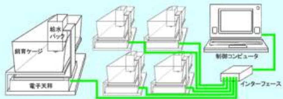
図2 装置概念図
