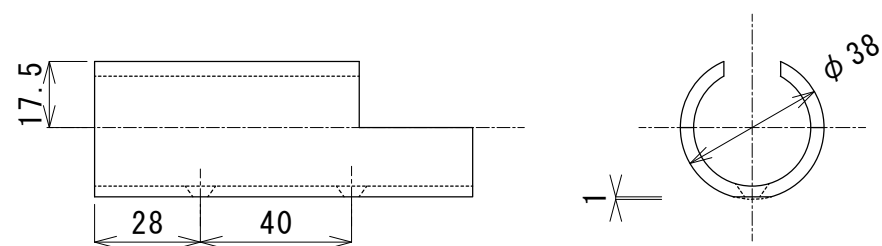
透明塩ビパイプVP30 内径31 外径38 肉厚3.5
