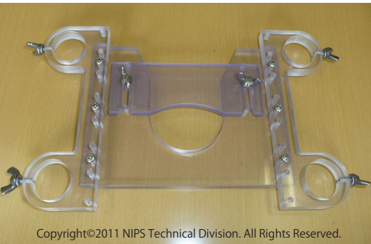
胴固定部
