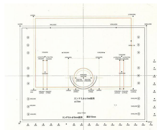
首固定部設計図
