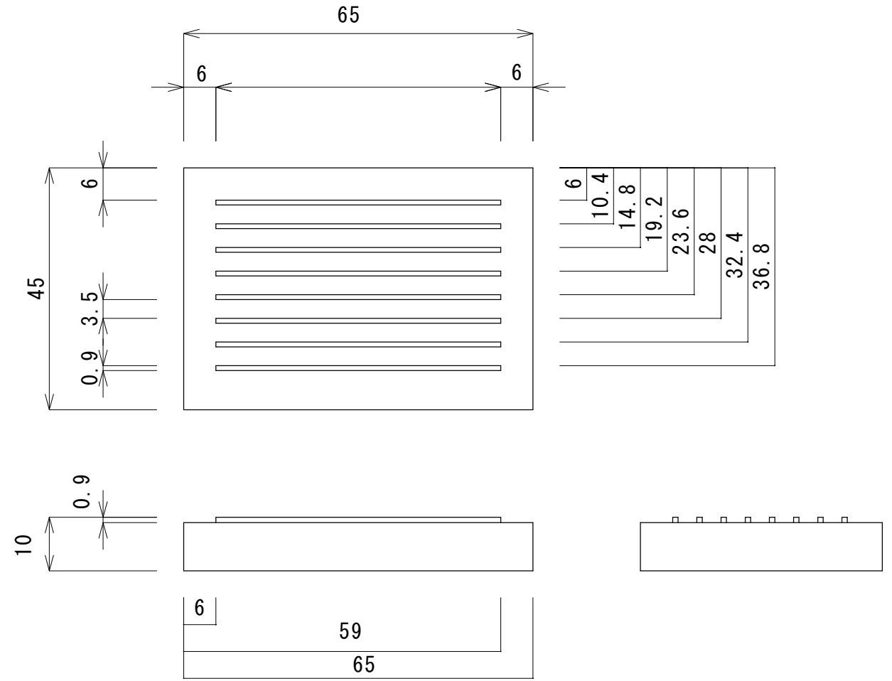
0.9mm の突起
