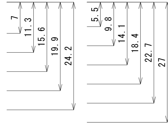
Vカッター中心 φ3エンドミル中心
