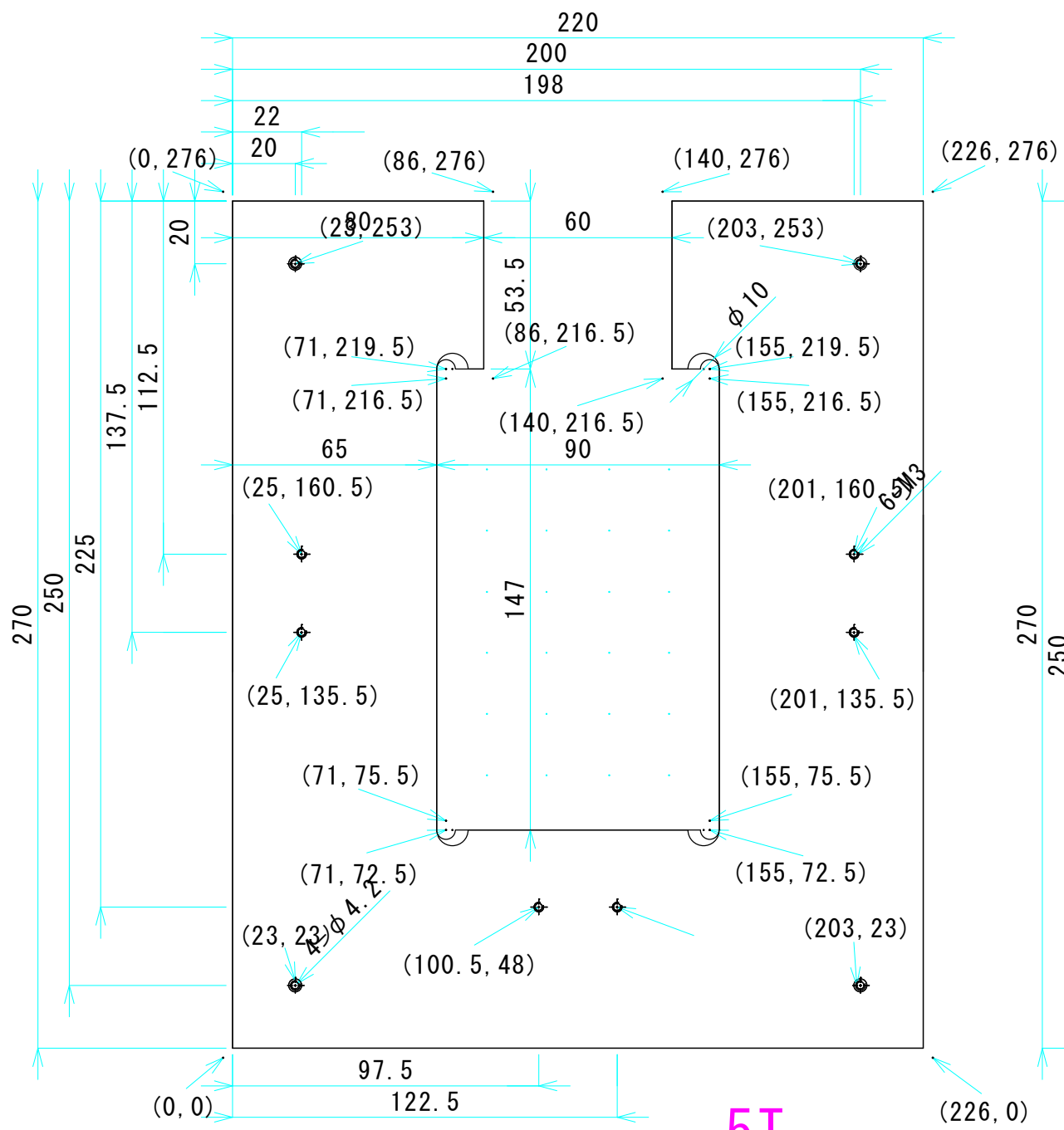
チェンバー底の センサー位置固定パーツ
