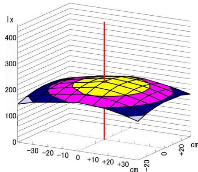
LED照明 2
