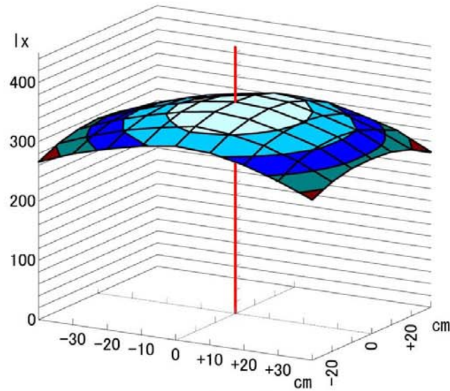
蛍光管
