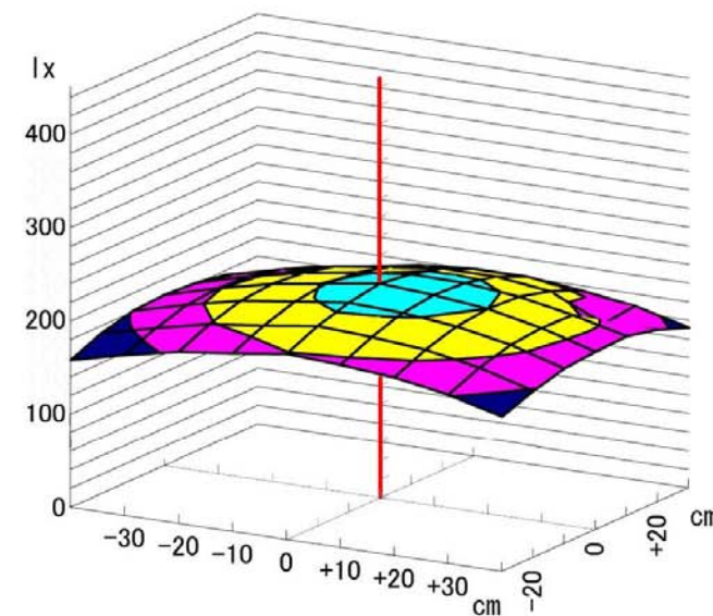
LED照明 3
